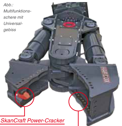
durchgehende Stahlschneide
